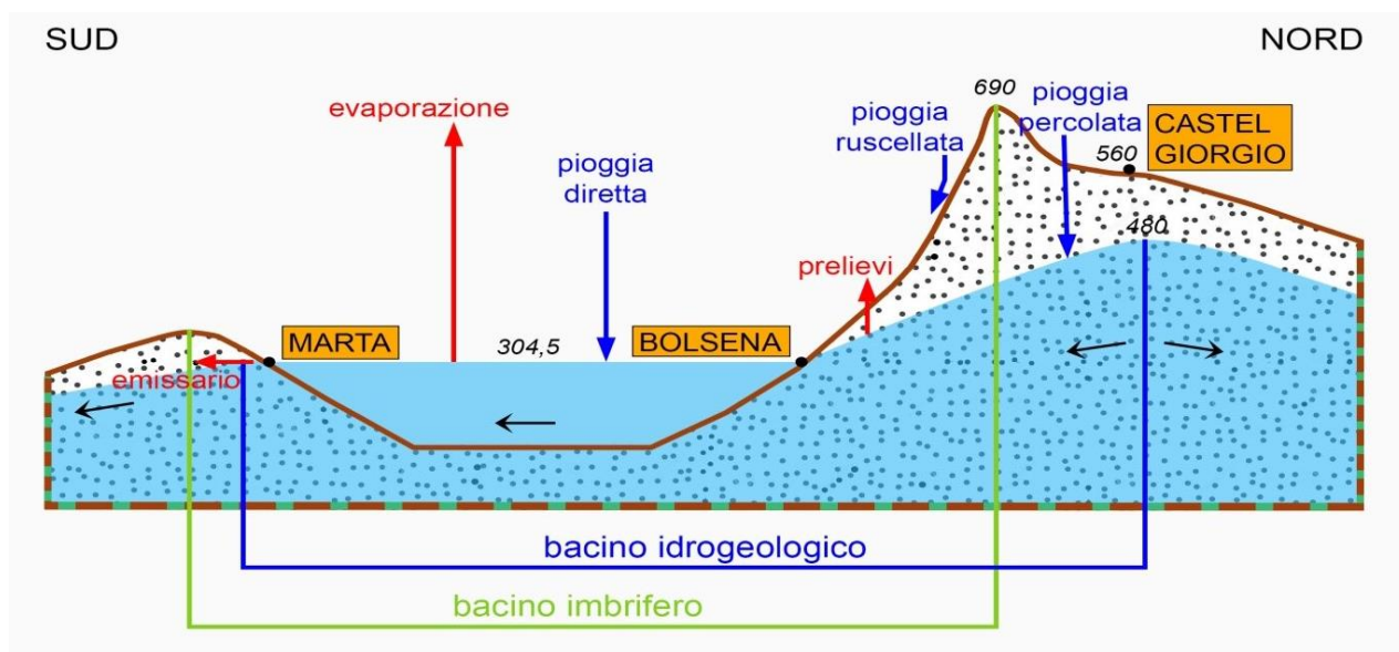
Schema dei flussi nella falda
